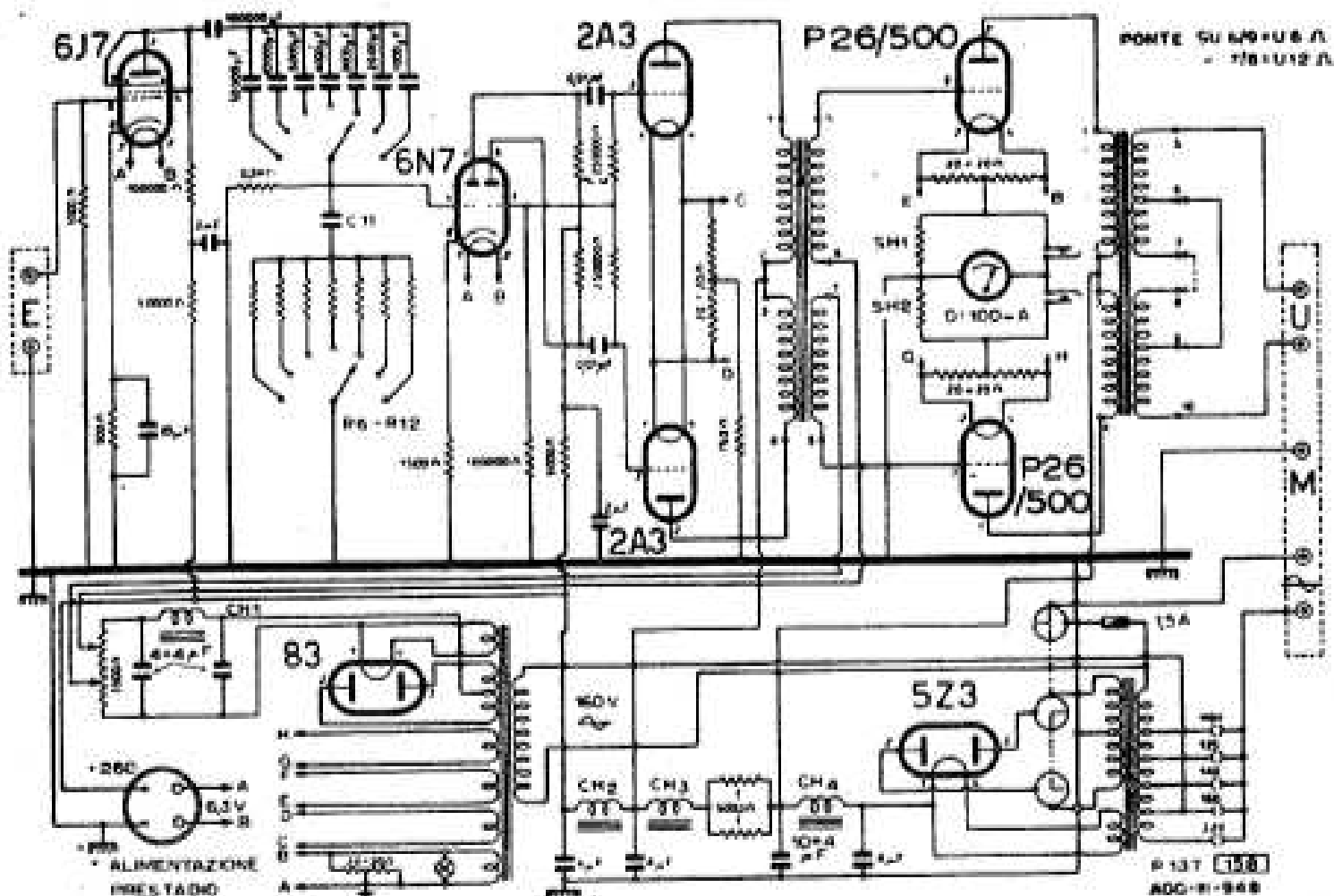
Allocchio Bacchini Amplificatore D 65 PN
